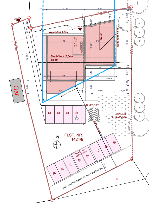
Grundriss UG 1:100
